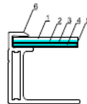
Section A-A 8:1
